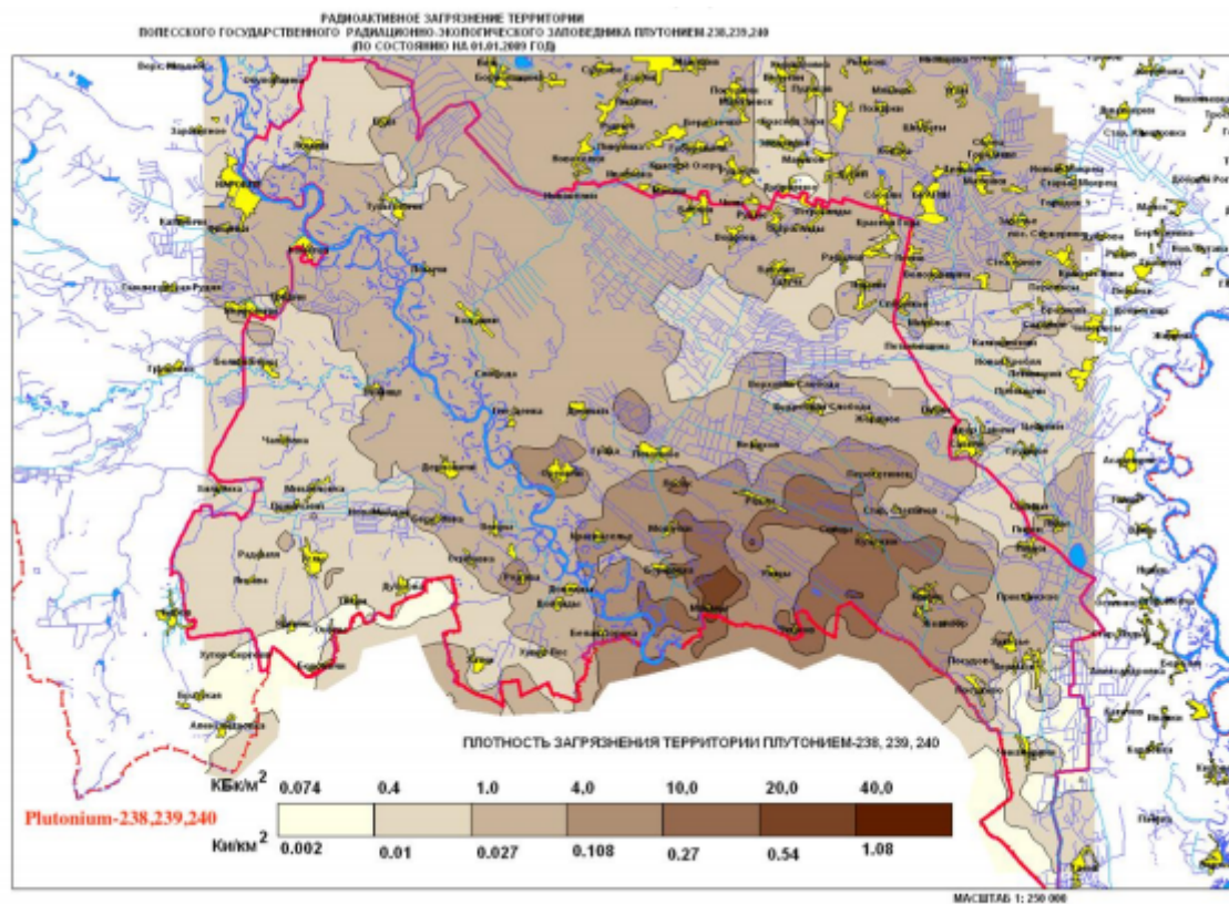
Рисунок А3: Карта 2009 г. осаднения плутония-238, 239, 240 на почве в белорусской части зоны отчуждения Чернобыльской АЭС. Верхняя шкала указана в КБк/м 2 , а нижняя шкала в Ки/км 2 .
