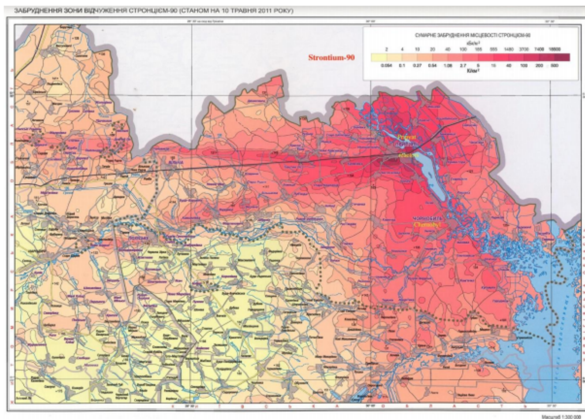
Рисунок А10: Карта осаждения стронция-90 на почве в украинской части зоны отчуждения Чернобыльской АЭС, 2011 г. Верхняя шкала указана в кБк/м 2 , а нижняя шкала в Ки/км 2 .
