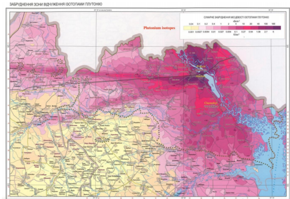
Рисунок А11: Карта осаднения изотопов плутония на почве в украинской части зоны отчуждения Чернобыльской АЭС, 2011 г. Верхняя шкала указана в \text{кБк}/\text{м}^2 , а нижняя шкала в \text{Ки}/\text{км}^2 .
