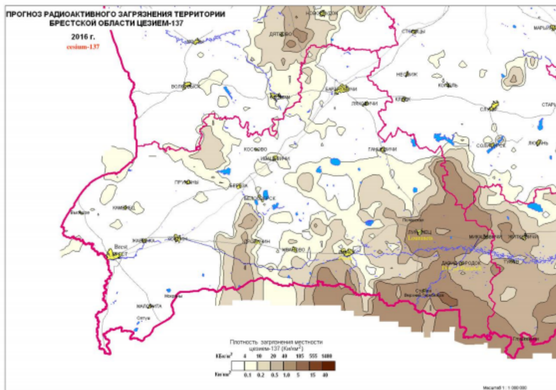
Рисунок А7: Карта 2016 г. осадения цезия-137 на почве в Брестской области. Верхняя шкала указана в \text{кБк}/\text{м}^2 , а нижняя шкала в \text{Ки}/\text{км}^2 .
