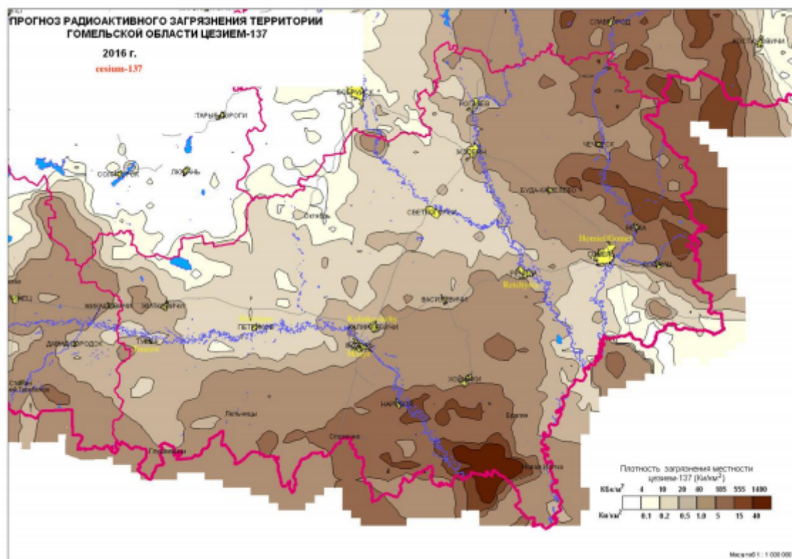
Рисунок А6: Карта 2016 г. осадения цезия-137 на почве в Гомельской области. Верхняя шкала указана в кБк/м², а нижняя шкала в Ки/км².
