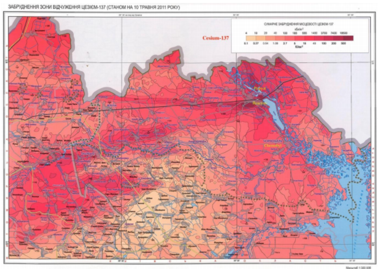
Рисунок А9: Карта осадения цезия-137 на почве в украинской части зоны отчуждения Чернобыльской АЭС, 2011 г. Верхняя шкала указана в \text{кБк}/\text{м}^2 , а нижняя шкала в \text{Ки}/\text{км}^2 .
