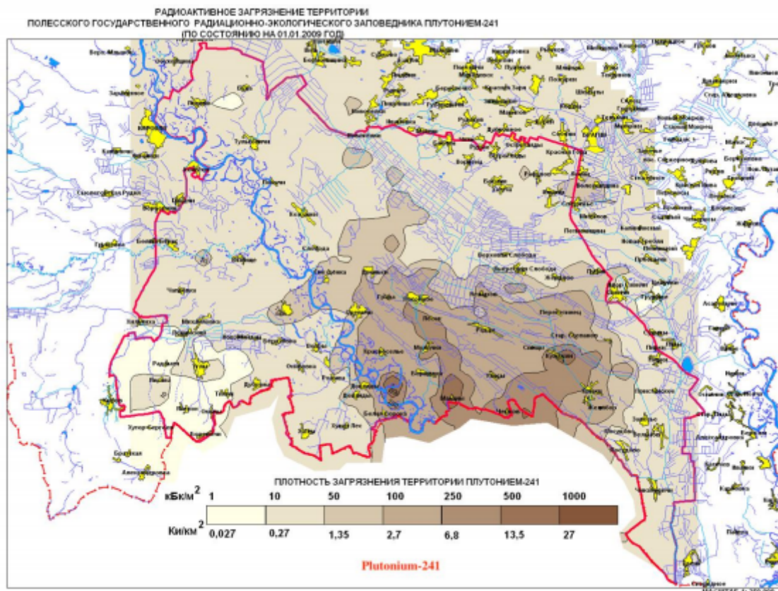
Рисунок А4: Карта 2009 г. осадения плутония-241 на почве в белорусской части зоны отчуждения Чернобыльской АЭС. Верхняя шкала указана в кБк/м 2 , а нижняя шкала в Ки/км 2 .
