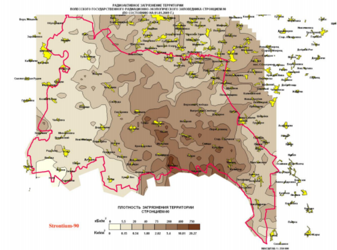
Рисунок А2: Карта 2009 г. осаднения стронция-90 на почве в белорусской части зоны отчуждения Чернобыльской АЭС. Верхняя шкала указана в \text{кБк}/\text{м}^2 , а нижняя шкала в \text{Ки}/\text{км}^2 .
