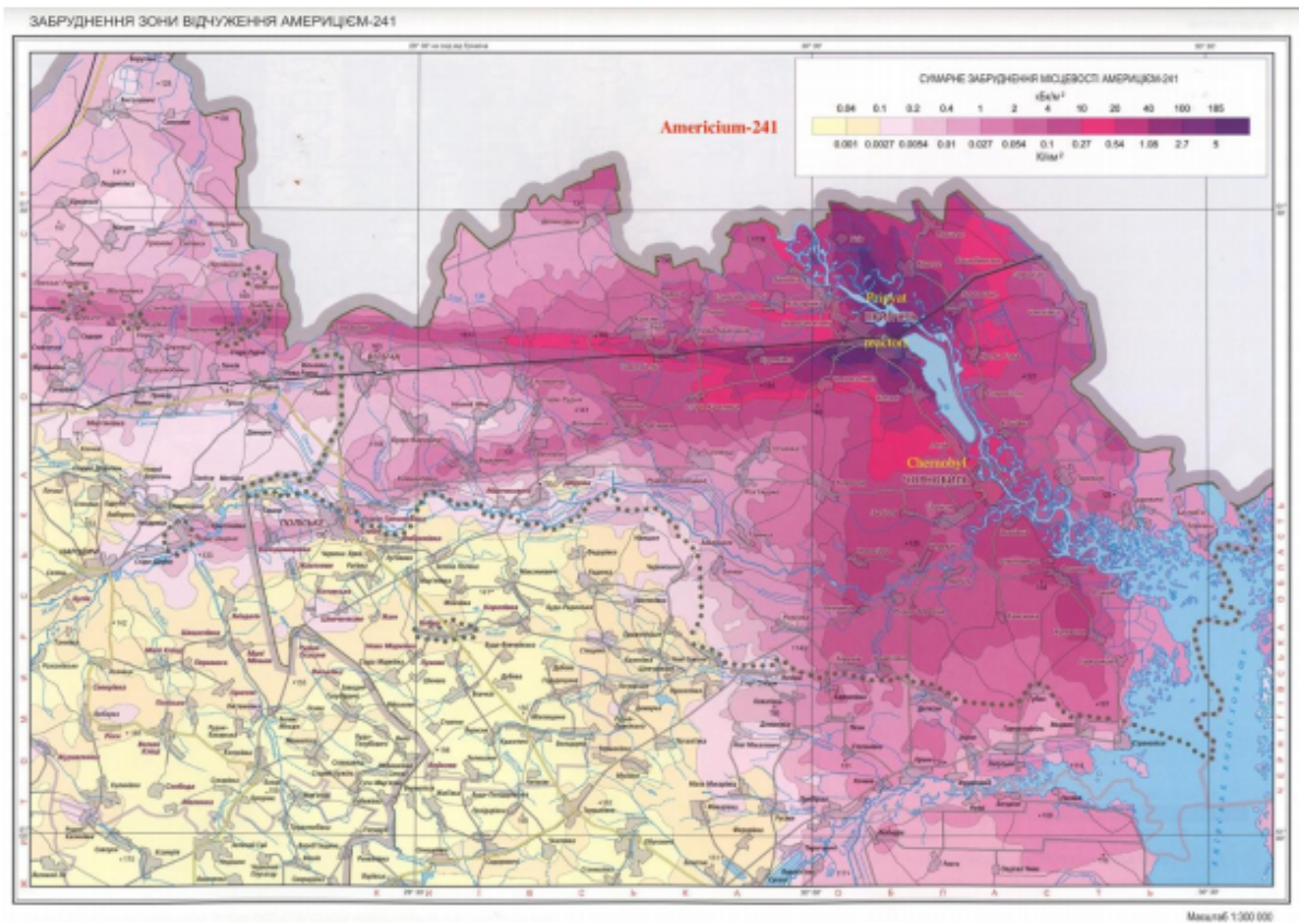
Рисунок А12: Карта осаждения америция-241 на почве в украинской части зоны отчуждения Чернобыльской АЭС, 2011 г. Верхняя шкала указана в кБк/м², а нижняя шкала в Ки/км².
